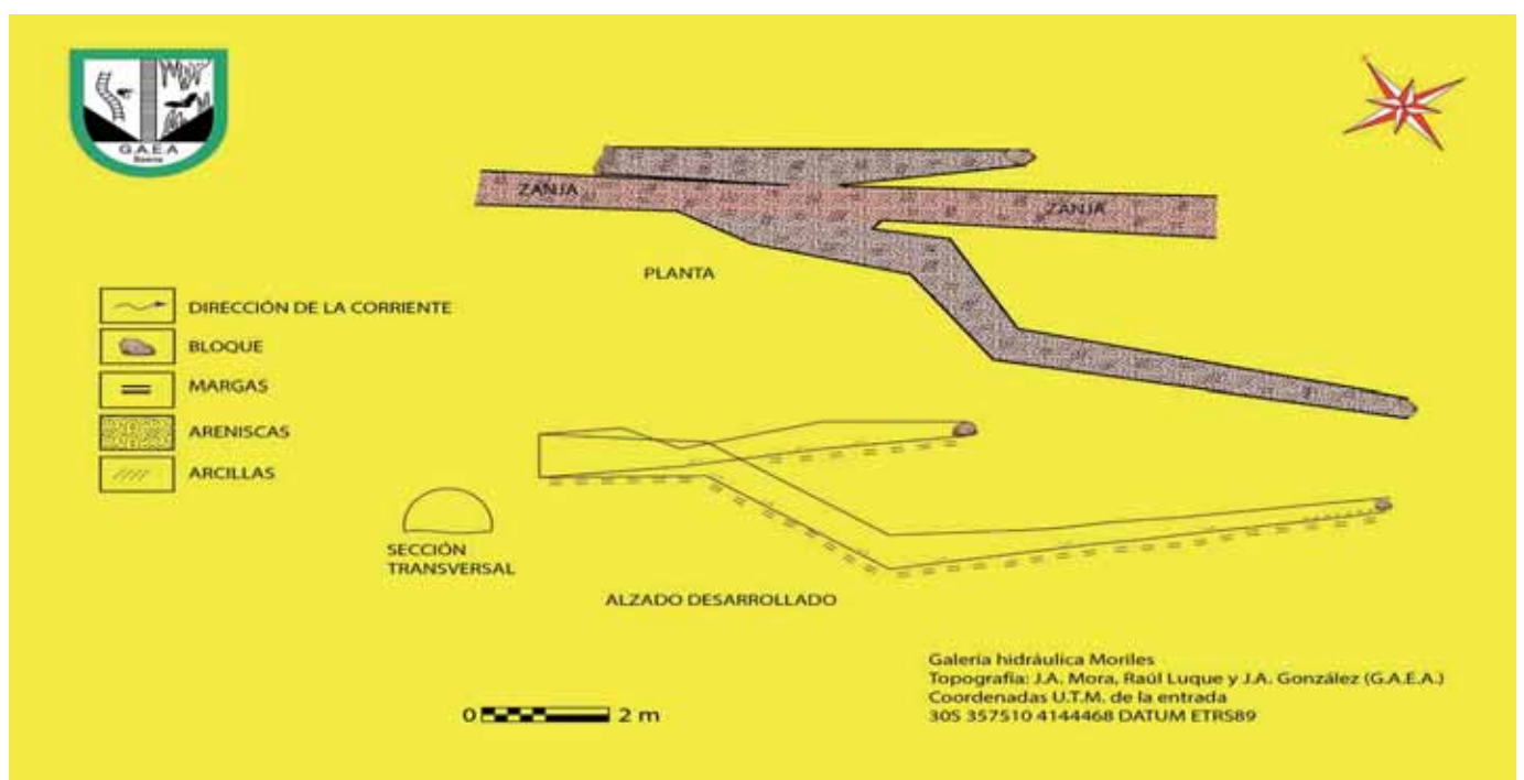
Figura 4: plano de la Galería hidráulica de Moriles.
